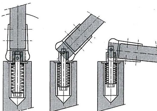
De werking van het scharnier.
