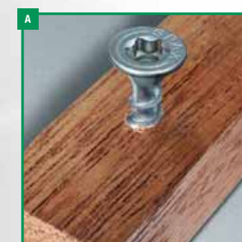
Afbeelding A: De SPAX® met 4CUT-punt: Zuiver indraaien, zonder dat het hout splijt.
