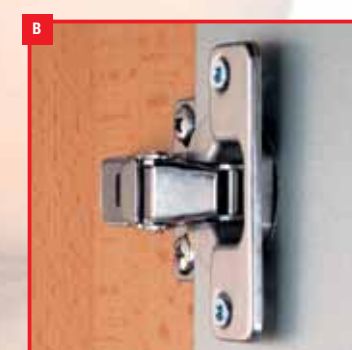
Afbeelding B: Een traditionele spaanplaatschroef: Ongereemd doordraaien van de schroef, het beslag zit niet vast.
