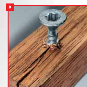
Afbeelding B: Een traditionele spaanplaatschroef: Splijten van het hout bij het indraaien.
