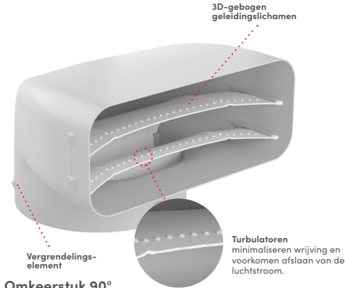
Omkeerstuk 90° P-UR 150 COMP-4051011
