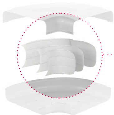
P-RBH 150 Buisbocht horizontaal 90° COMP-4051006
