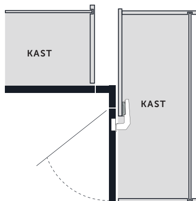
Minimale voeg F voor fronten met frontradius (R = 1 mm) bij nul-instelling
