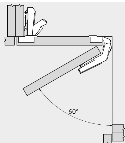
De top van het vouwdeurscharnier wordt in dezelfde front gemonteerd als de top v/h 170°- respectievelijk 155°-scharnier
